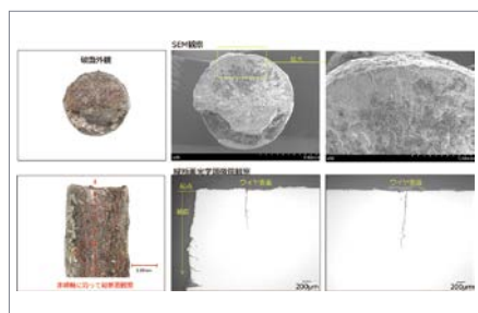
破面観察
