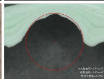
断面計測
