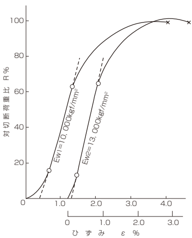
図 7.27 平行よりIWRC 6×37グループ (静素用・Pr=8.0Dr)
