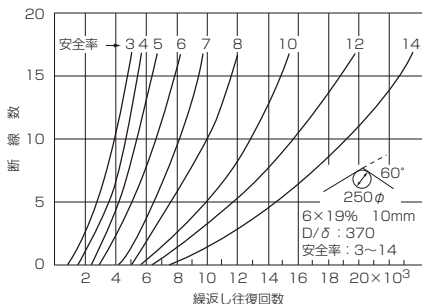
図 7.6 安全率の影響
