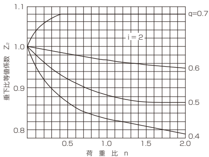
付図 2.2 垂下比等値係数算出図(2 荷重)
