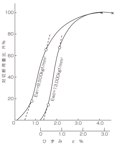
図 7.24 平行よりIWRC 6×19グループ (動素用・Pr=6.3Dr)
