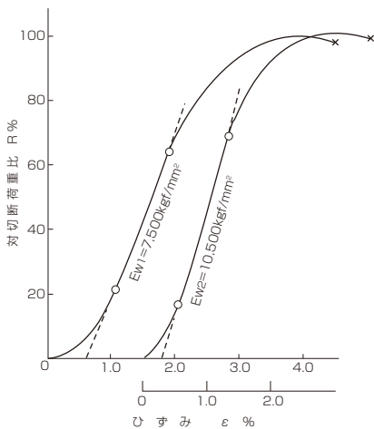
図 7.19 6 × 24 O/O (Pr=6.7Dr)
