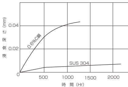
図 6.15 595℃過熱水蒸気中の腐食
