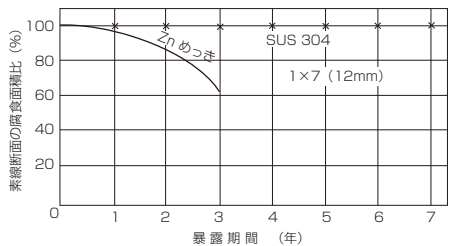
図 6.13 腐 食 度
