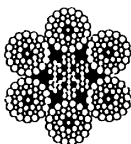
IWRC 6 \times SWS(49)
