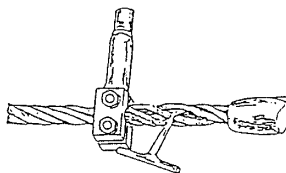
端末金具に近いロープ末端における内部点検 (無張力)
