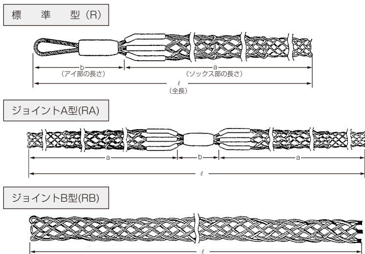
■TYPE-R標準寸法表
