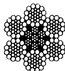
IWRC 6 \times WS(31) (JIS)
