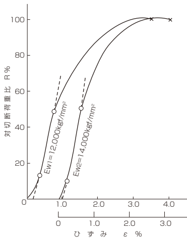
図 7.29 7 × 7 G/O (Pr=8.0Dr)
