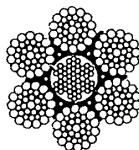
DF IWRC 6 x WS (36)
