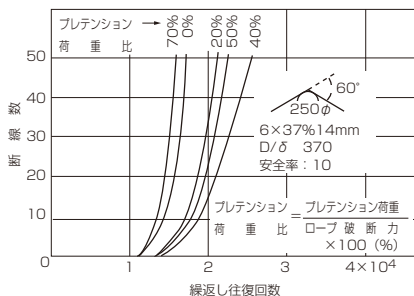
図7.4 プレテンションの影響
