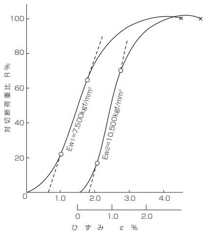
図 7.21 6×61 O/O( Pr=6.7Dr )
