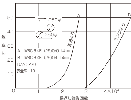
図7.1 普通よりとラングよりの比較
