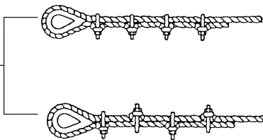
図 5.1 グリップ法の止め方
