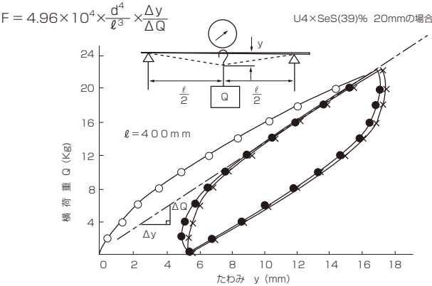
図 7.10 横荷重一たわみ曲線
