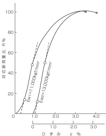
図 7.31 7 × 19 G/O (Pr=8.0Dr)
