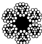
6 x F{(3 x 2 + 3) + 12}
