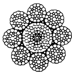
DF IWRC 8 x P-WS (36)
