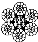
IWRC 6 × P · WS (26)
