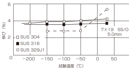
図 6.19 低温におけるロープの伸び
