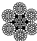
IWRC 6 x SeS (37)
