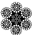
IWRC 6 \times WS(36) (JIS)
