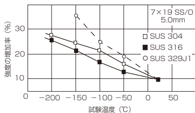
図 6.18 低温におけるロープの強度
