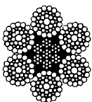
IWRC 6 \times WS(41) (JIS)
