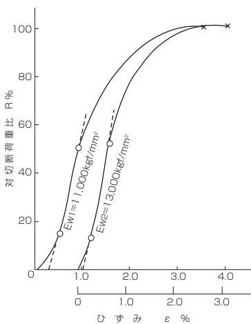
図 7.28 7 × 7 G/O (Pr=6.7Dr)
