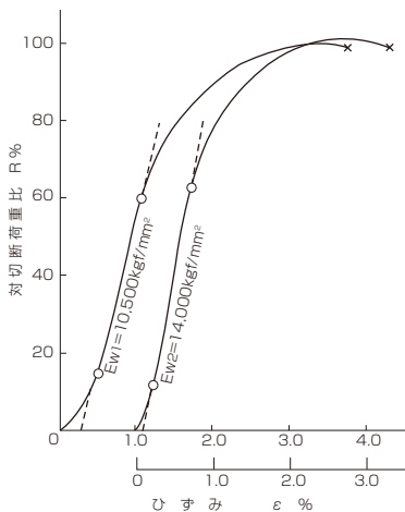
図 7.37 平行よりCFRC 6×37グループ (静索用・Pr=8.0Dr)
