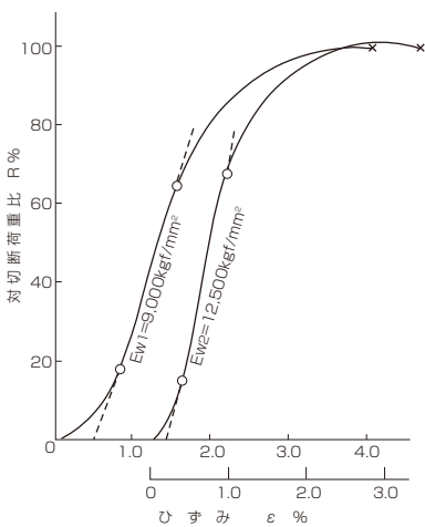
図 7.26 平行よりIWRC 6×37グループ (動素用・Pr=6.3Dr)
