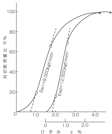
図 7.22 平行より 6×19グループ( Pr=6.3Dr )
