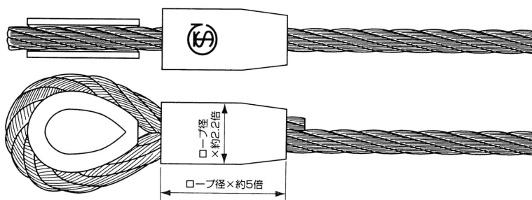
アイロック®の形状
