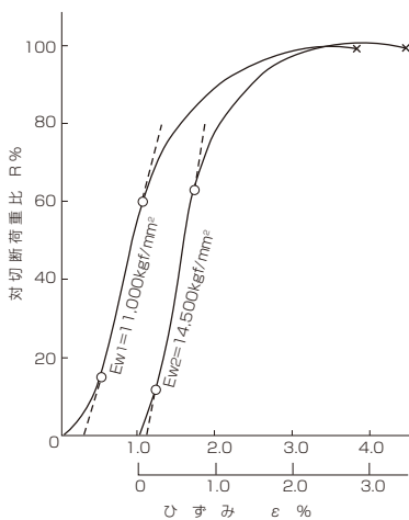
図 7.35 平行よりCFRC 6×19グループ (静素用・Pr=8.0Dr)
