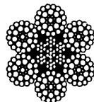
IWRC 6 \times SFi(41)
