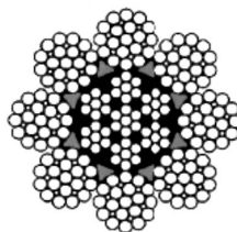
図 4. 7 オメガフィラー®ロープの断面図例 (OF IWRC 8×Fi(25))
