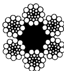
6 \times WS(26) (JIS)
