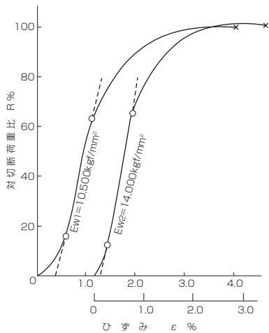
図 7.25 平行よりIWRC 6×19グループ (静素用・Pr=8.0Dr)
