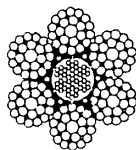
DF IWRC 6 x Fi (29)
