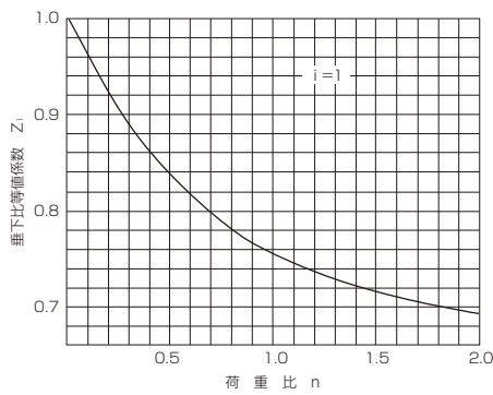
付図 2. 1 垂下比等価係数算出図(1 荷重)
