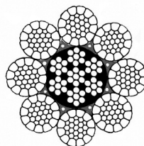
図 4. 5 デルタフィラーロープの断面図例 (DF-G IWRC 8×WS(31))
