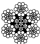
IWRC 6 \times WS(26) (JIS)
