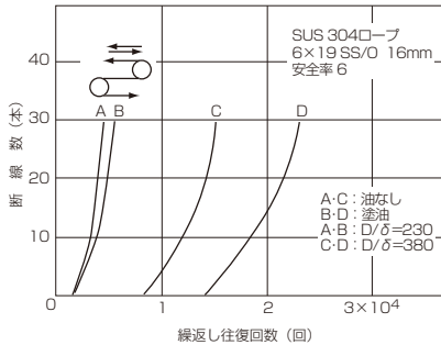
図 6.4 塗油の影響
