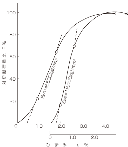
図 7.18 6 × 19 O/O (Pr=6.7Dr)
