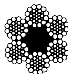
6 \times WS(31) (JIS)
