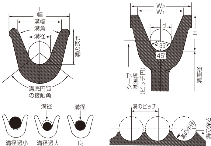
図 8.1 シープ及びドラムの溝寸法
