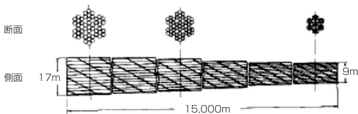
図 4. 9 テーパードロープ構造例
