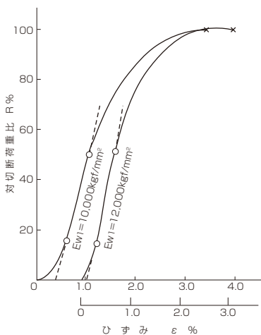
図 7.30 7 × 19 G/O (Pr=6.7Dr)
