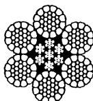
IWRC 6 × P · WS (31)
