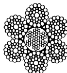
DF IWRC 6 x WS (41)
