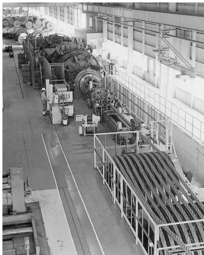
製網機(クローザ)
