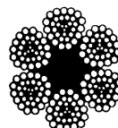
6 x F{(3 x 2 + 3) + 12 + 15}
