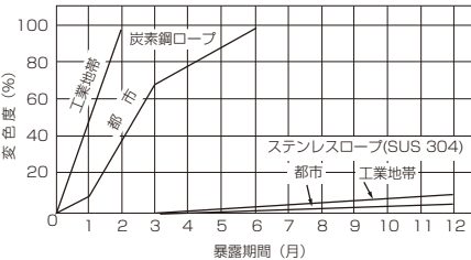
図 6. 7 大気中における変色
