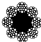
8 x W (19) (JIS)
