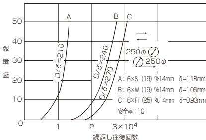
図 7.5 D/dの影響
