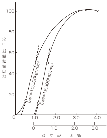
図 7.33 7×37 G/O(Pr=8.0Dr)
