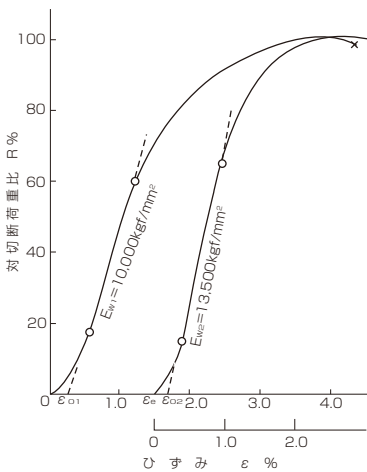
図 7.16 6 × 7 C/L (Pr=7.75Dr)
