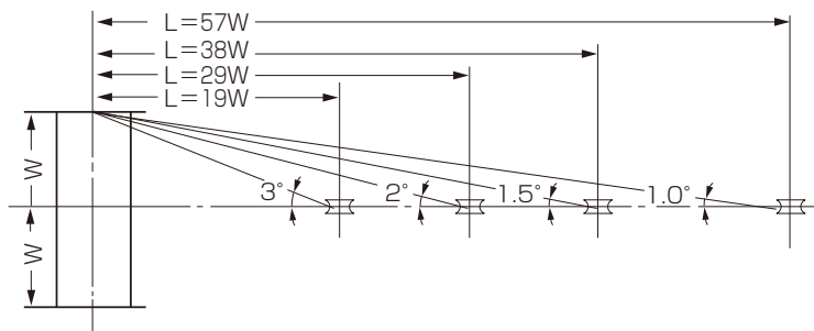
図 8.3 フリートアングル
