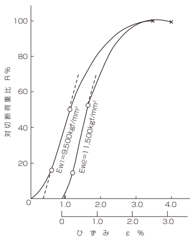
図 7.32 7×37 G/O(Pr=6.7Dr)
