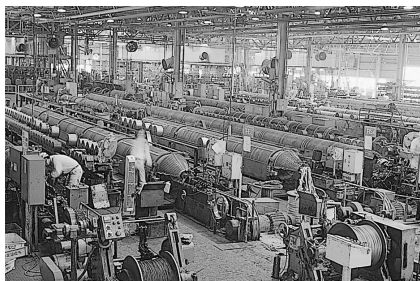
より線機(ストランダ)
