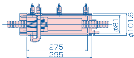
1S21.8W-CS型接続具
