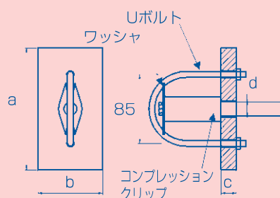
TCUL型定着具
